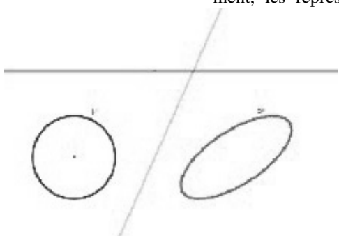
Un cercle et son image obtenue comme trajectoire d'un point-image.
